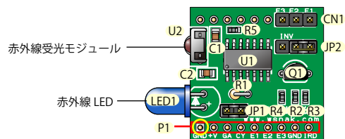
#286 赤外線発光 / 受光ボード
