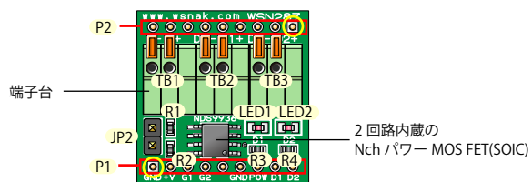
#287 2ch FET ボード
