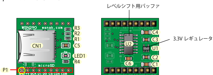
#290 μSD カードボード
