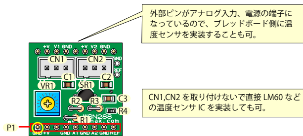
#288 温度センサ / ショントレギュレータ
